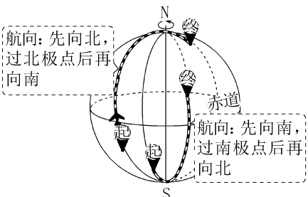
c. 两地分别位于南、北半球 注意：若图中起点和终点互换，则航向不变。
