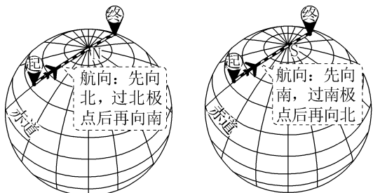
a. 两地同位于北半球 注意：若图中起点和终点互换，航向还是先向北，过北极点后再向南。 b. 两地同位于南半球 注意：若图中起点和终点互换，航向还是先向南，过南极点后再向北。
