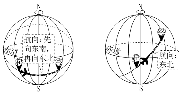
c. 两地位于南半球同一纬度 注意：若图中起点和终点互换，则航向为先向西南，再向西北。 d. 两地分别位于南、北半球 注意：若图中起点和终点互换，则航向为西南（相反方向）。
