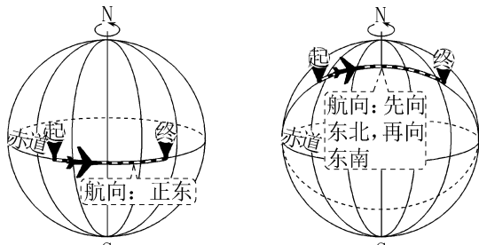
a. 两地同在赤道上 注意：若图中起点和终点互换，则航向为正西。 b. 两地位于北半球同一纬度 注意：若图中起点和终点互换，则航向为先向西北，再向西南。
